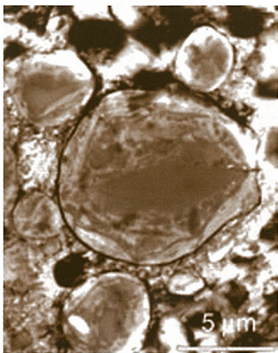
Fig. E. Microfósiles de microorganismos criptoendolíticos embebidos en jarosita (color claro) encontrados en las rocas de Mount Fleming, Valles Secos, Antártida. Algas y hongos coloreados artificialmente.
