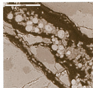
Fig. C. Imagen de microscopía electrónica indicando la presencia de hongos y algas dentro de las fisuras de rocas Antárticas.
