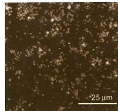
Fig. D. Imagen de microscopía láser confocal con marcaje específico LIVE/DEAD mostrando células de bacterias endolíticas vivas y muertas.
