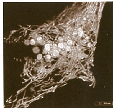
Fig. B. Reconstrucción tridimensional de un protoliquen endolítico ocupando un poro de arenisca, compuesto por células algales (células redondas) y células fúngicas (células alargadas).
